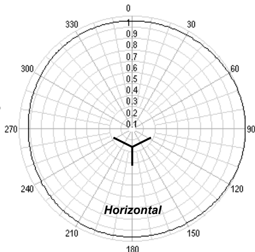
Diagramas Radiação (98 MHz - Cpol) @ anel TTFM3A escala E/Emáx
